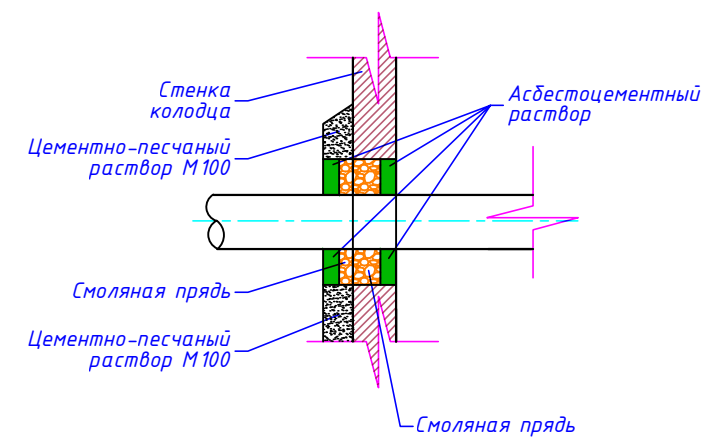
Узел "А"
