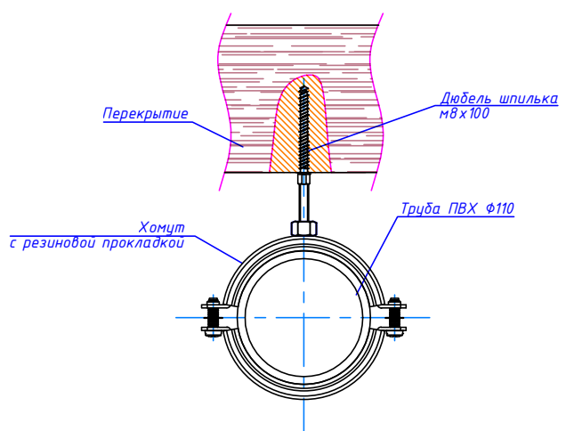
Узел крепления трубопроводов
