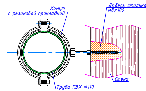
Узел крепления трубопроводов
