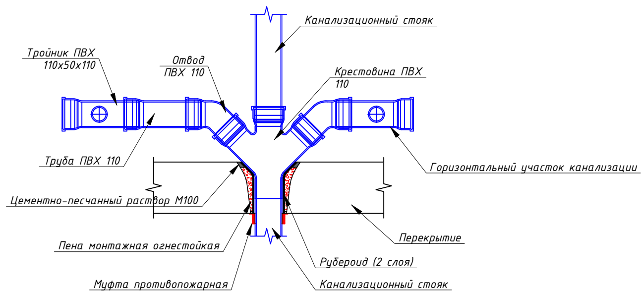
Пропуск канализационного стояка через перекрытие
